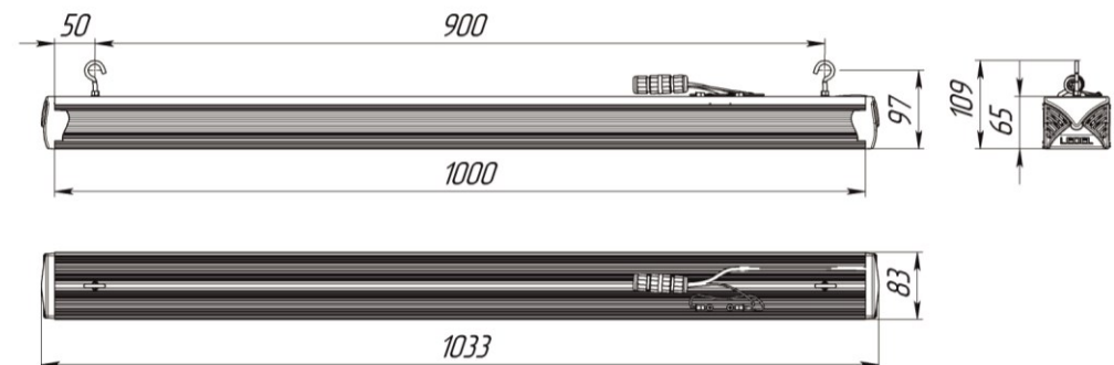
Рисунок 2 Светильник «L-industry NEW 48, L-industry NEW 48Т». Подвесной вариант
