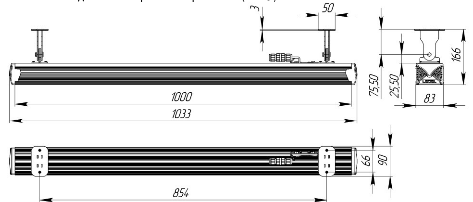
Рисунок 1 Светильник «L-industry NEW 48, L-industry NEW 48Т». Поворотный вариант
